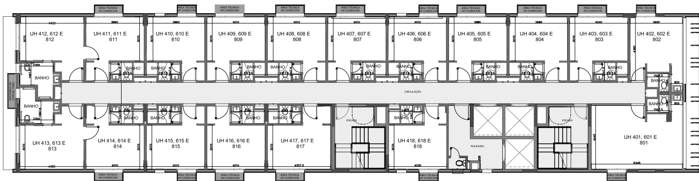
N PLANTA BAIXA 04º, 06º E 08º PAVIMENTO
