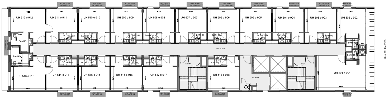
N PLANTA BAIXA 05° E 09° PAVIMENTO
